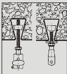
Spojovací prvky závěsů HOLOCLIP a HOLOBAR
